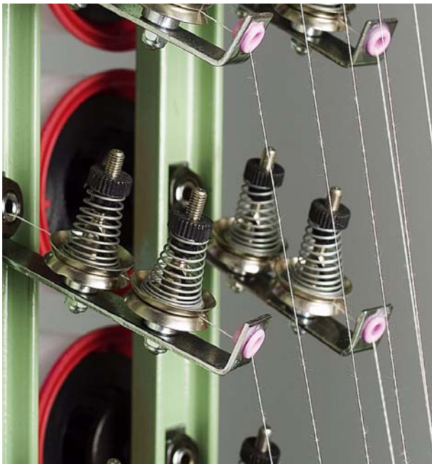
每根纱线张力通过线刹单独可调
