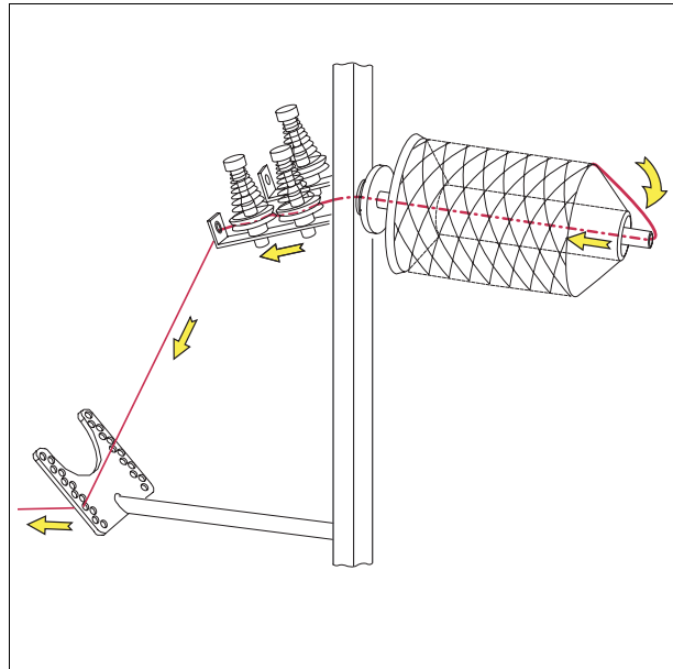
从筒子喂纱的简图
