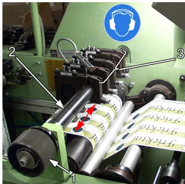
Schneidbalken mit seitlicher Verstellung
