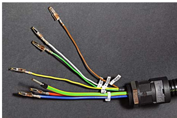
电线卷曲接触连接至控制盒
