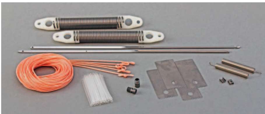
用于MBJ3.0 MK-12-05199 纬纱输送装置和选色装置的组件
