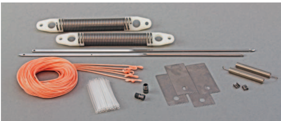
Juego de piezas para transporte de trama y mando de colores para MBJ3.0 MK-12-05199
