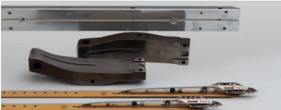
Juego de repuestos para modificación de pinzas de MBJ3.0 a MBJ3.1, sin compensación neumática de la trama y sin VARISPEED (Entrega mínima) MK-12-05216 (con compensación neumática de la trama: MK-12-06240)
