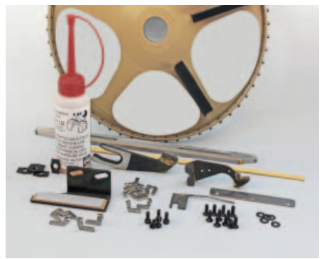
Juego de piezas para mecanismo de tisaje de MBJ3.0 MK-12-05198
