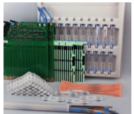
Juego de repuestos para máquina Jacquard SPE MBJ3.0 MK-12-05200
