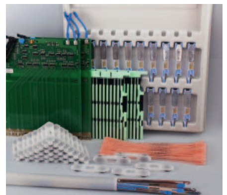
Kit pièces de rechange machine Jacquard pour SPE MBI3.0 MK-12-05200
