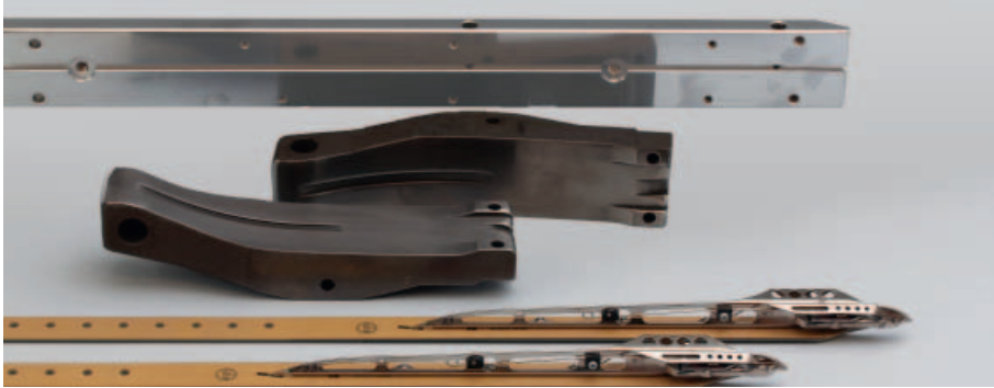
Kit pièces de rechange pour changement de pince de la MBJ3.0 pour passage en MBJ3.1 sans compensation pneumatique fil de trame et sans VARISPEED (étendue de livraison minimum) MK-12-05216 (avec compensation pneumatique fil de trame: MK-12-06240)
