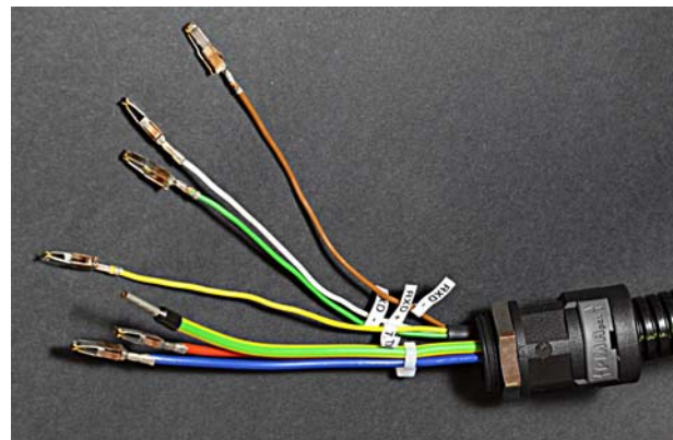
电线卷曲接触连接至控制盒
